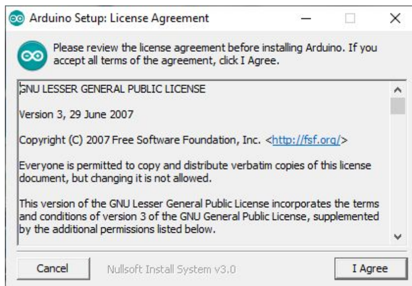
fig. 6.2.3.2 - Arduino Lizenzbedingungen
